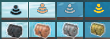
Harpon basique
